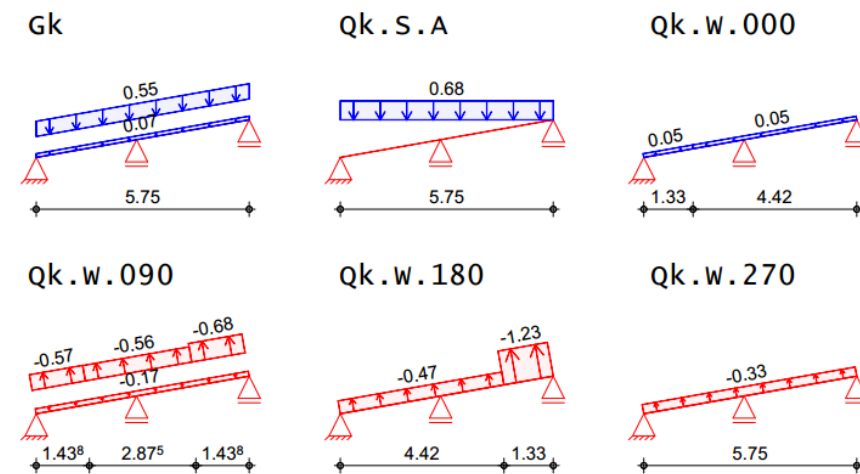
Belastungsgrafiken (Einwirkungsbezogen)
